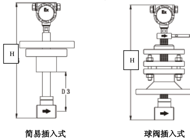
图四 插入式传感器结构示意图
