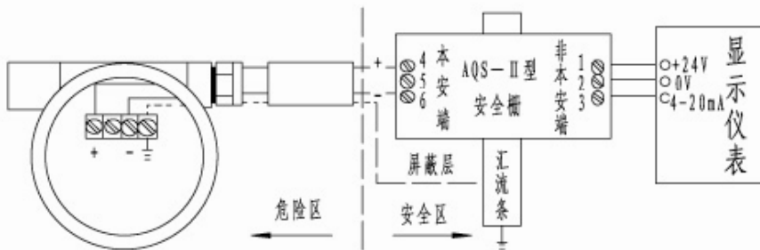
压力变送器配AQS-II型齐纳安全栅接线方法
