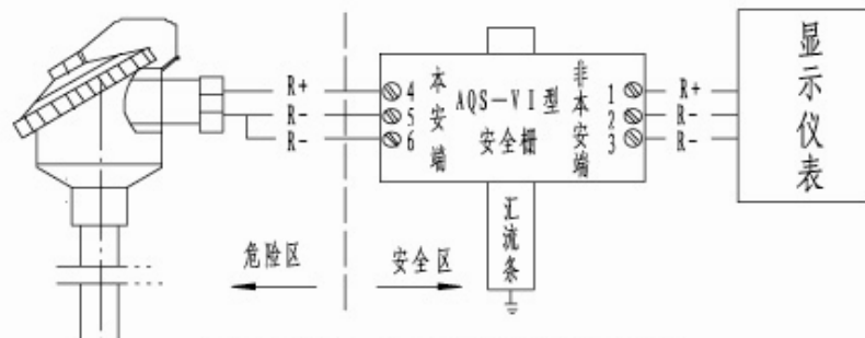
热电阻配AQS-VI型齐纳安全接线方法
