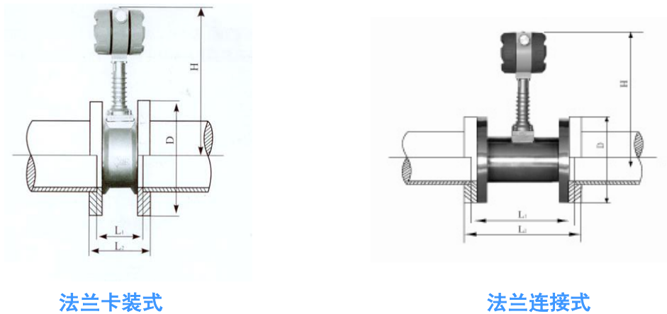
图三 法兰卡装式和法兰连接式外形尺寸示意图
