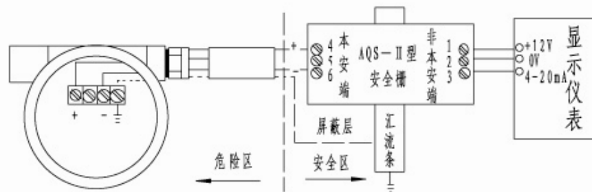
二线制电流输出流量变送器配AQS-II型齐纳安全栅接线方法
