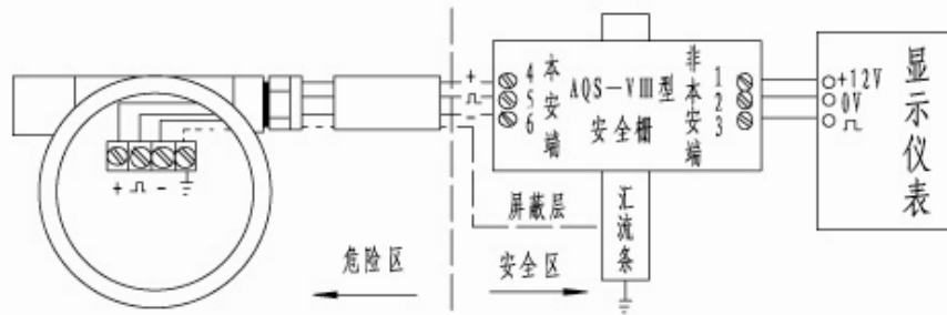
三线制脉冲输出流量传感器配AQS-VIII型齐纳安全栅接线方法
