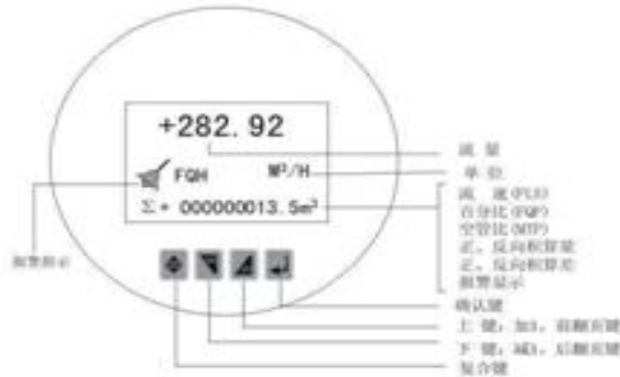
图.1 键盘定义与液晶显示
