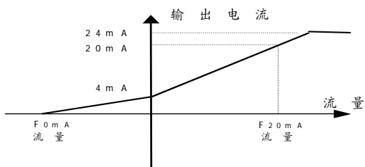
0 - 4 - 20 m A 方式输出特性
